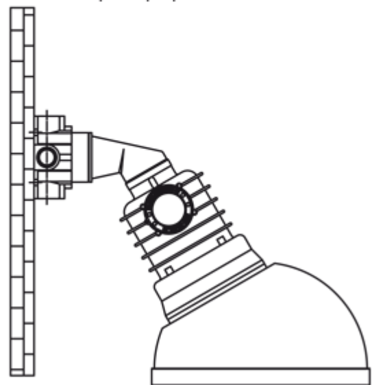
Пример крепления на стене
