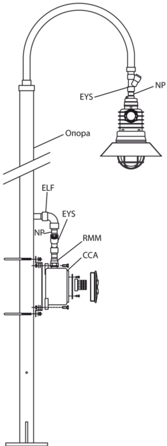
Пример крепления на мачте
